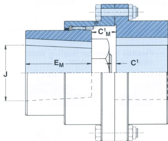
Flex-Rigid
