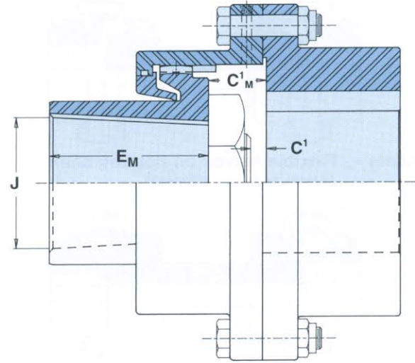
Flex-Rigid
